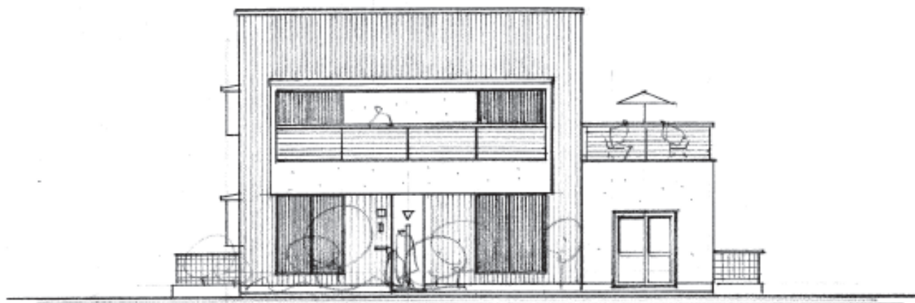
南立面図 SC=1/100
