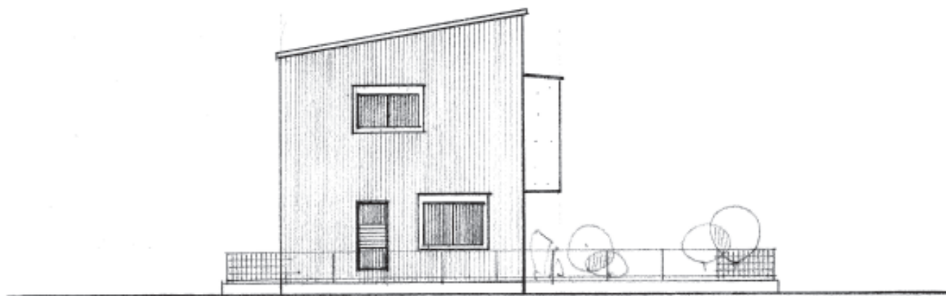
南立面図 SC=1/100
